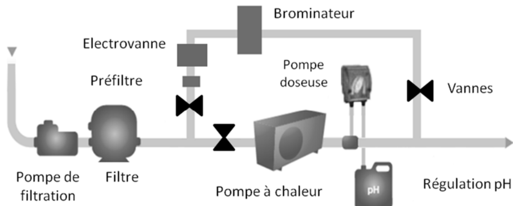
Figure 27. 1 ère possibilité d'installation du kit « régulation brome »
