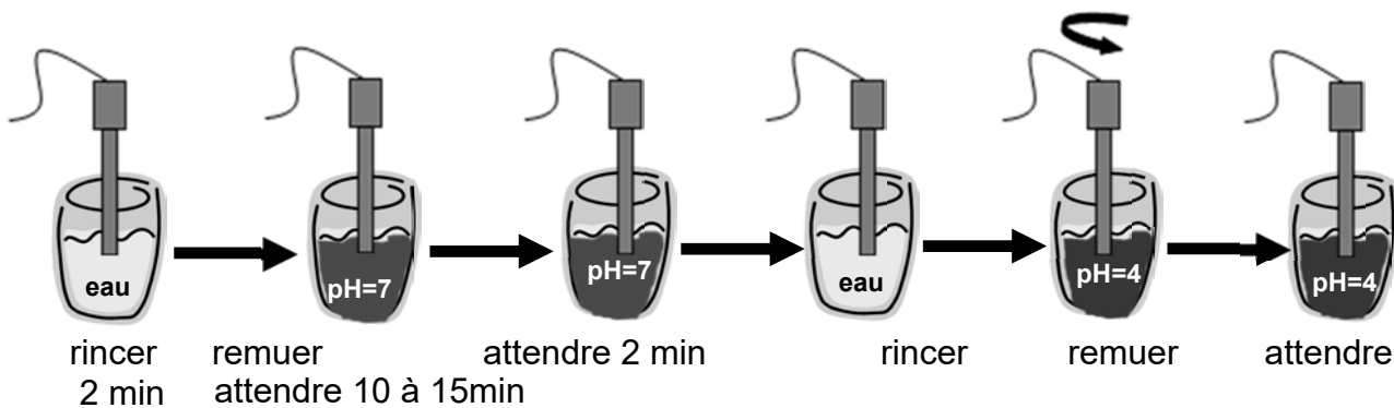
Figure 78. Calibration de la sonde pH
