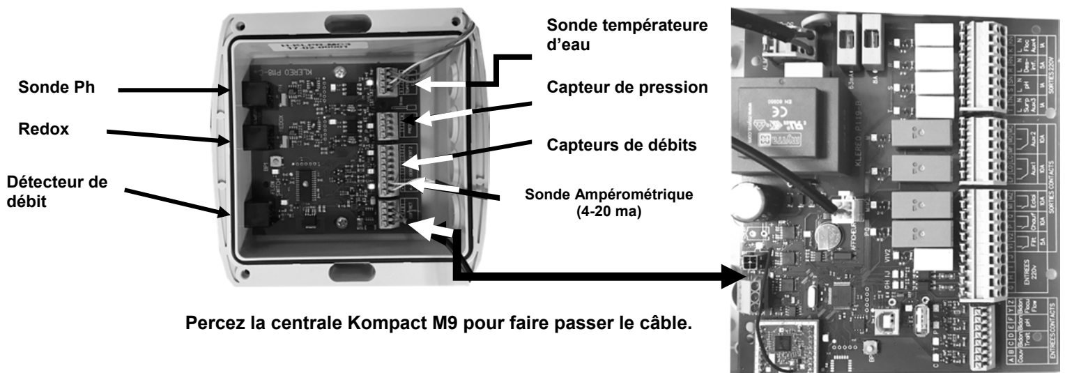
Figure 38. Raccordement de la centrale au boîtier multicapteurs
