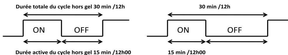
Figure 66. Possibilités de fonctionnement de la filtration en mode hors-gel
