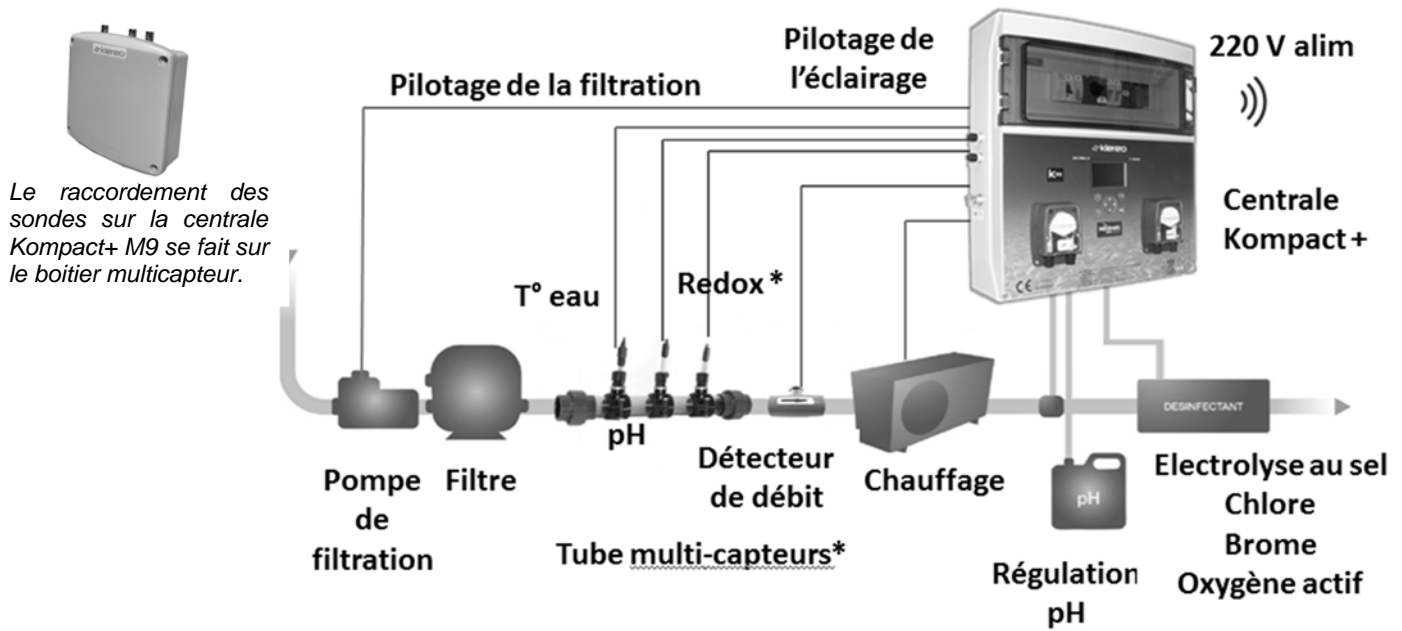
Figure 10. Diagramme d'installation Kompact +
