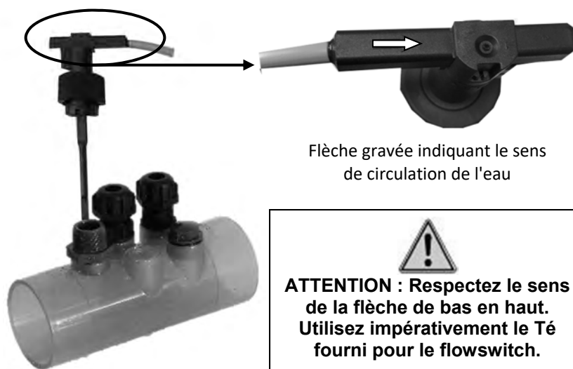
Figure 18. Montage du détecteur de débit
