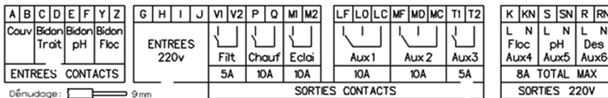
Figure 34. Entrées sorties de la carte centrale Kompact+M5
