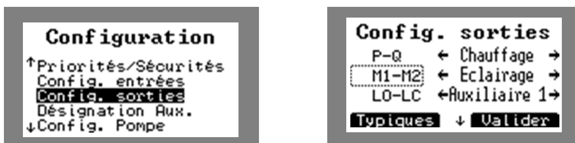
Figure 67. Configuration des sorties pour le Kompact M9
