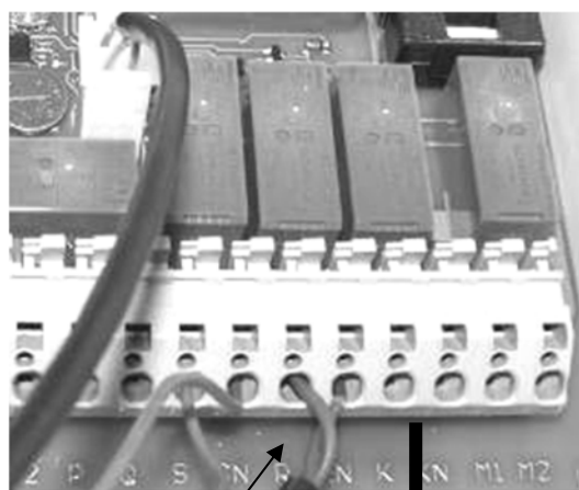
Figure 42. Branchement de l'alimentation de l'électrolyseur Klereo
