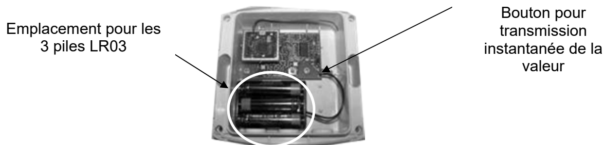
Figure 45. capteur température air
