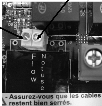
Figure 41. Câblage de l'alimentation de la cellule
