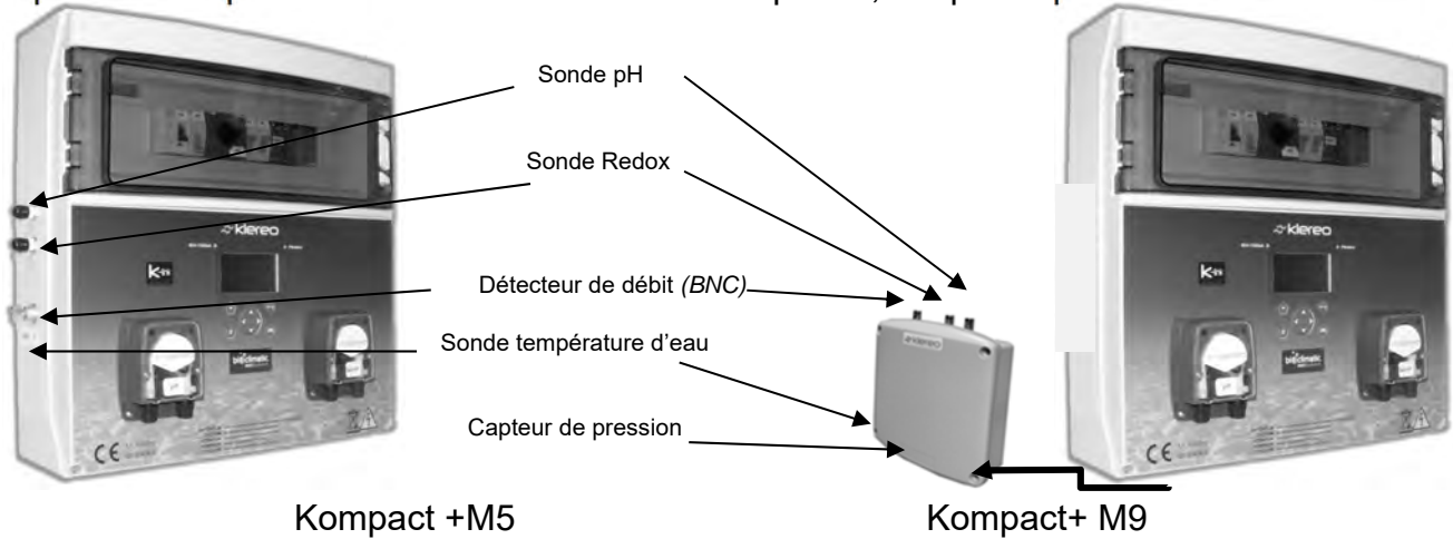
Figure 30. Branchement des capteurs sur la centrale Kompact +
