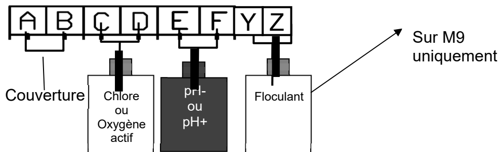
Figure 46. Branchements des détecteurs de fin de bidon
