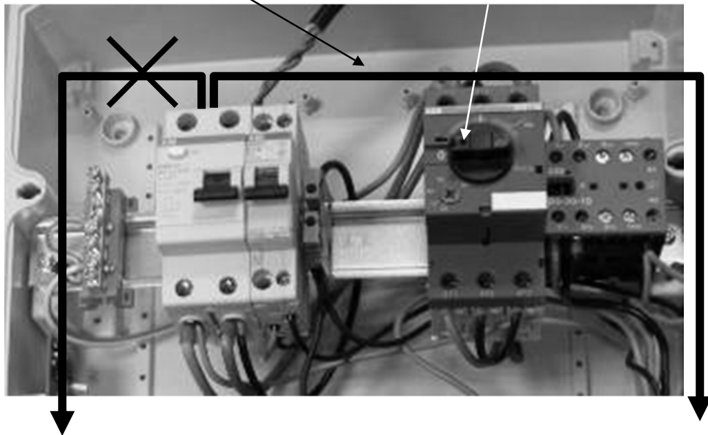
Figure 32. branchement de l'alimentation électrique du coffret Klereo Kompact +
