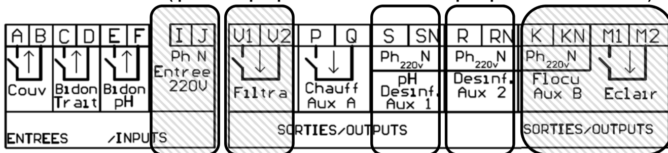
Figure 34. Entrées sorties de la carte centrale Kompact+M5
