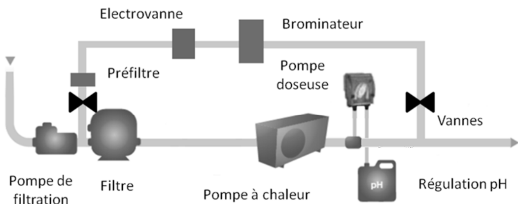
Figure 28. 2 ème possibilité d'installation du kit « régulation brome »
