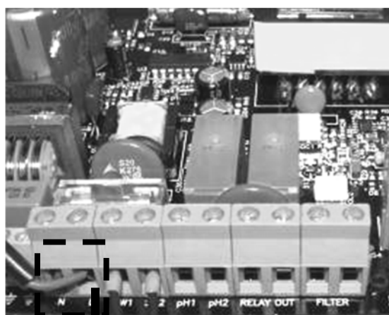
Figure 42. Branchement de l'alimentation de l'électrolyseur Klereo
