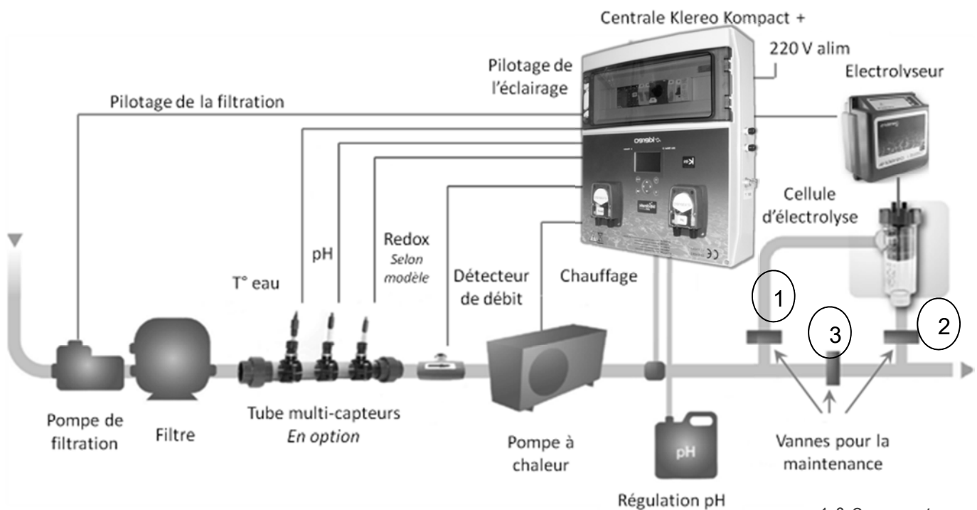
Figure 29. Installation de la cellule d'électrolyse
