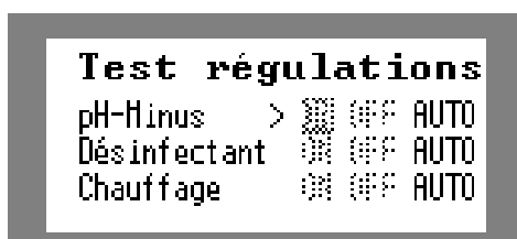
Figure 55. écran de test des régulations
