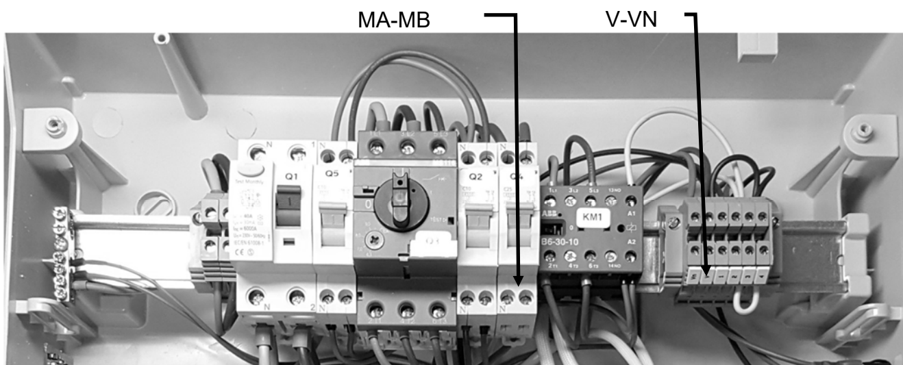
Figure 36. Intérieur du coffret Kompact +
